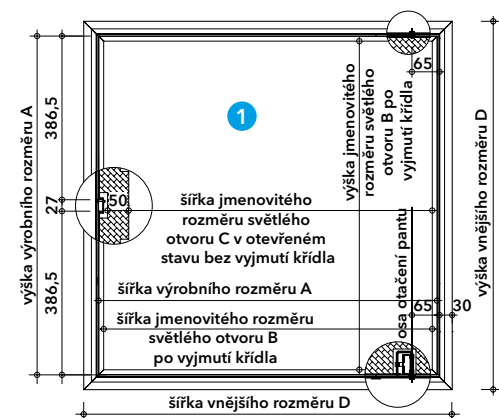
Detail A - rozměry
