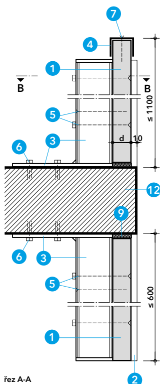
řez A-A
