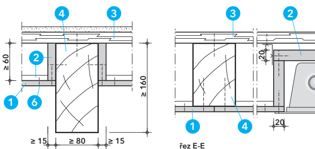
Detail J - varianta s viditelnými dřevěnými trámy - REI 30
