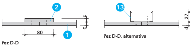
Detail I - překrytí spoje desek
