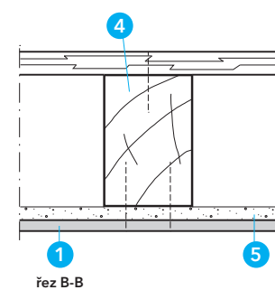
Detail C - opláštění pod omítnutými stropy
