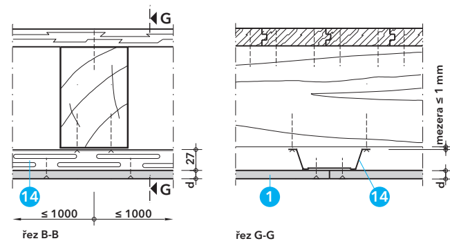
Detail G - připevnění na pružné lišty
